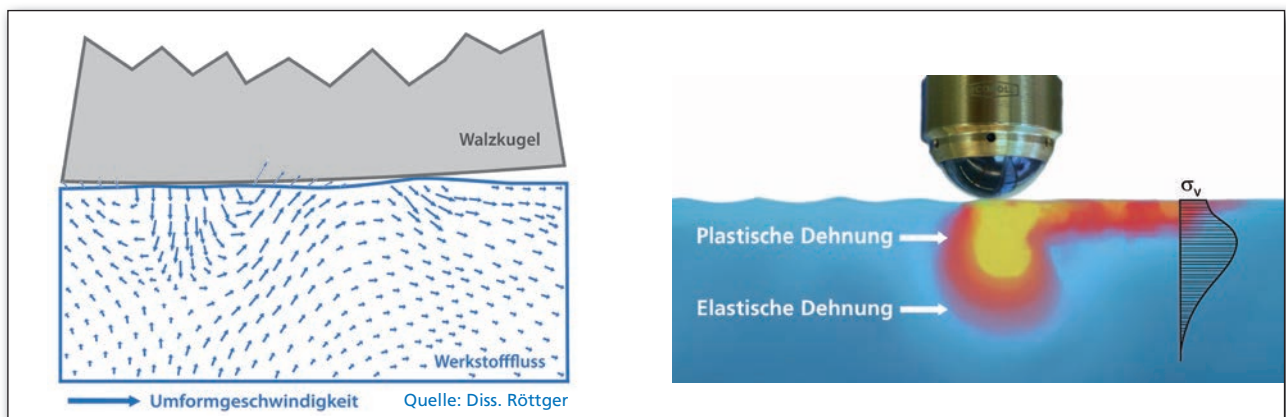
Bild 1: Randschichtumformung
