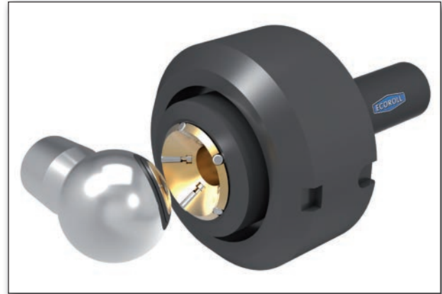
Glattwalzen einer Kugel mit Typ RKAK
